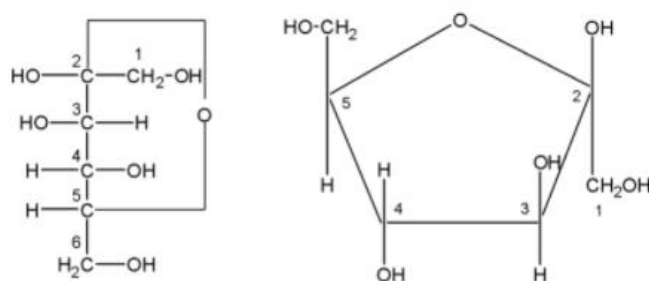
β-D-Fructose
