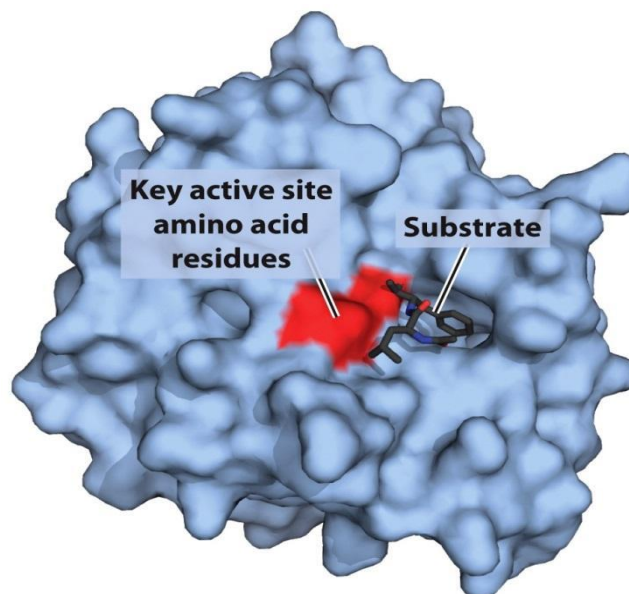
Fig. 5 Active Site Chymotrypsin
