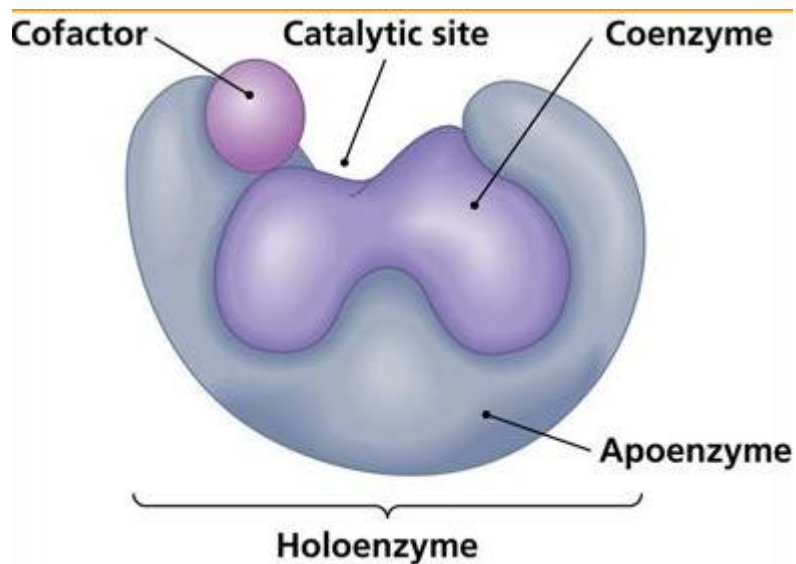
Fig. 4 Holoenzyme
